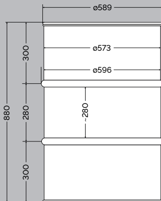
Standard-Stahlsackfässer (DS/EN 210).
