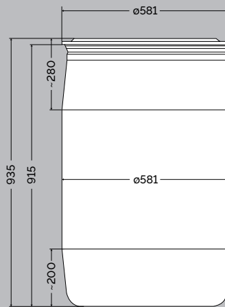
Standard-Kunststofffässer (DS/EN 12707).
